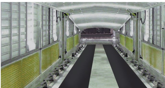
BCP-HPR rutschhemmende, selbstklebende Fahrstreifen bei geschlossenen Autotransportwaggons (ohne Radfeststeller)
